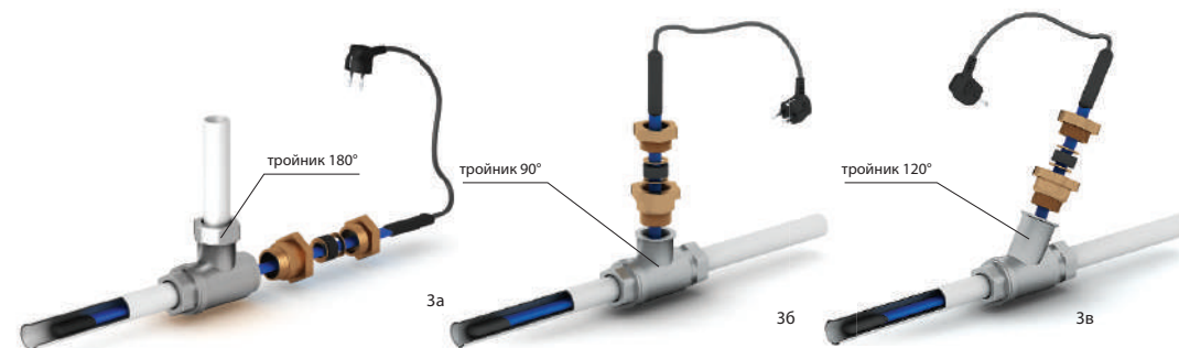
Рис.3. Схемы ввода нагревательной секции внутри трубопровода: а - прямой ввод; б - ввод под углом 90°; в - ввод под углом 120°
